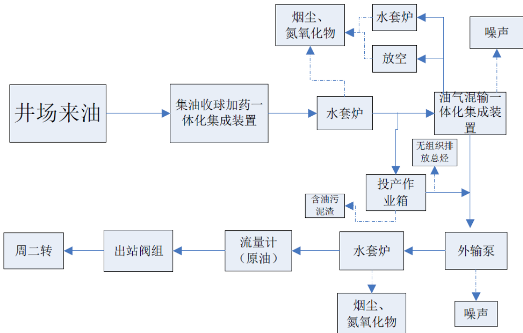
图 3-1 原油集输工艺流程及产污环节图
